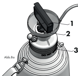
Kolbenstange nicht verriegelt
