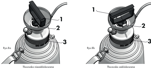
Tłocznisko niezablokowane
